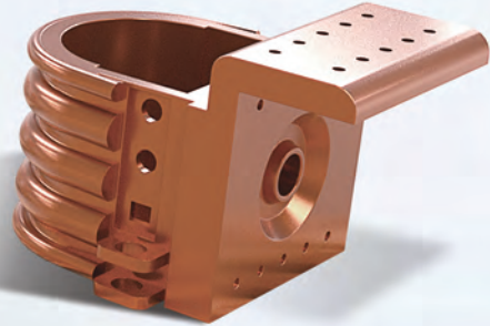
电极夹： 由高导电性铜制成， 电导率高于77%
