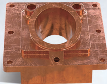
氧枪支架： 由高导电性铜制成， 电导率高于77%
