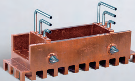
电器元件： 由高导电性铜制成， 电导率高于77%
