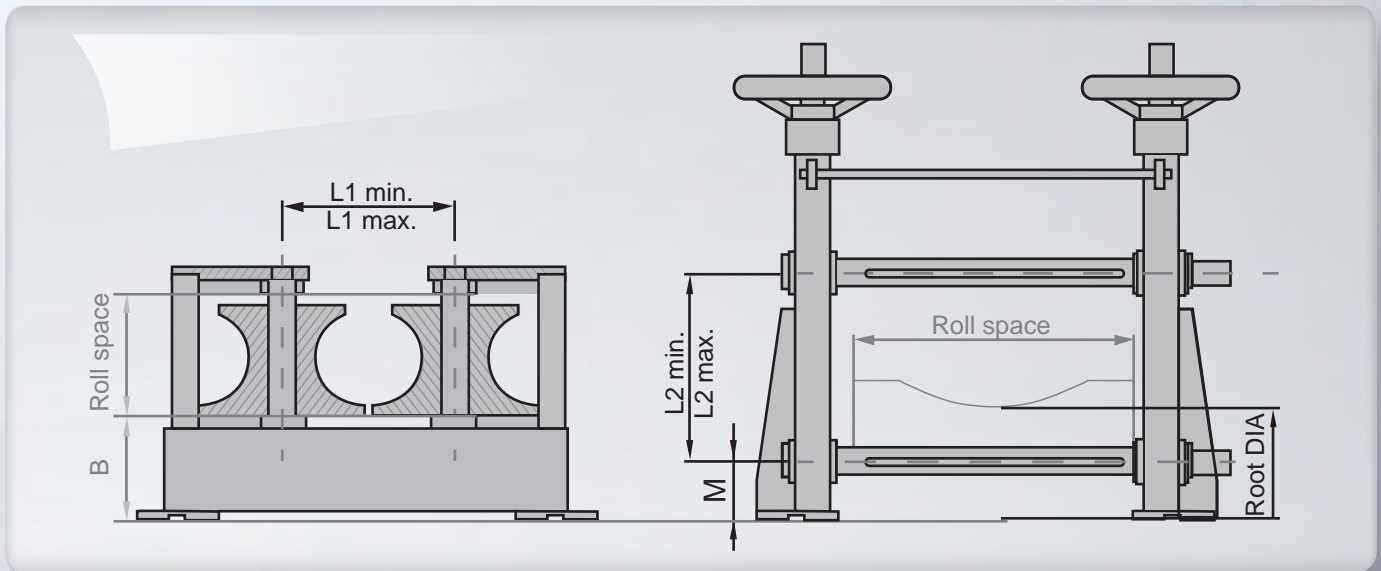
Vertikales Walzgerüst
